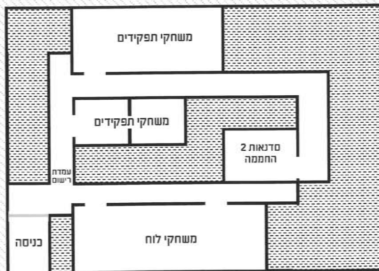
קומת מרתף (לא נגישה לנכים)
